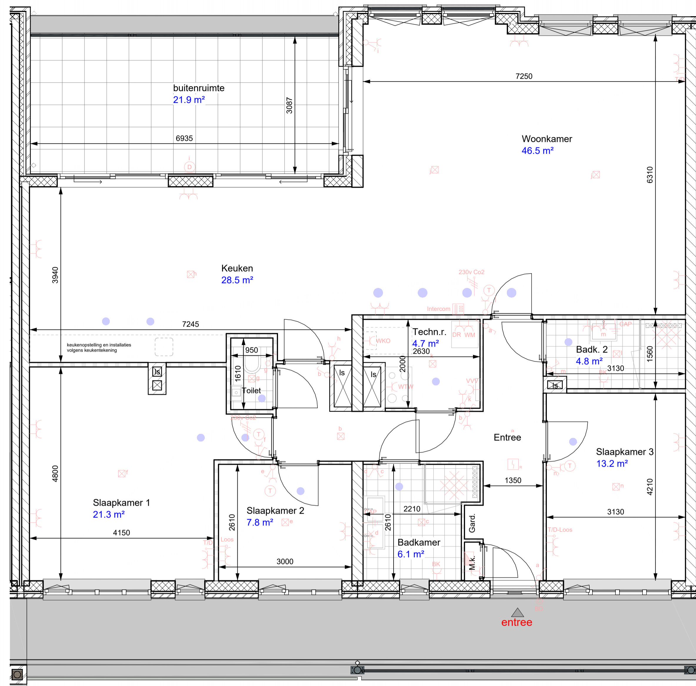
Plattegrond
